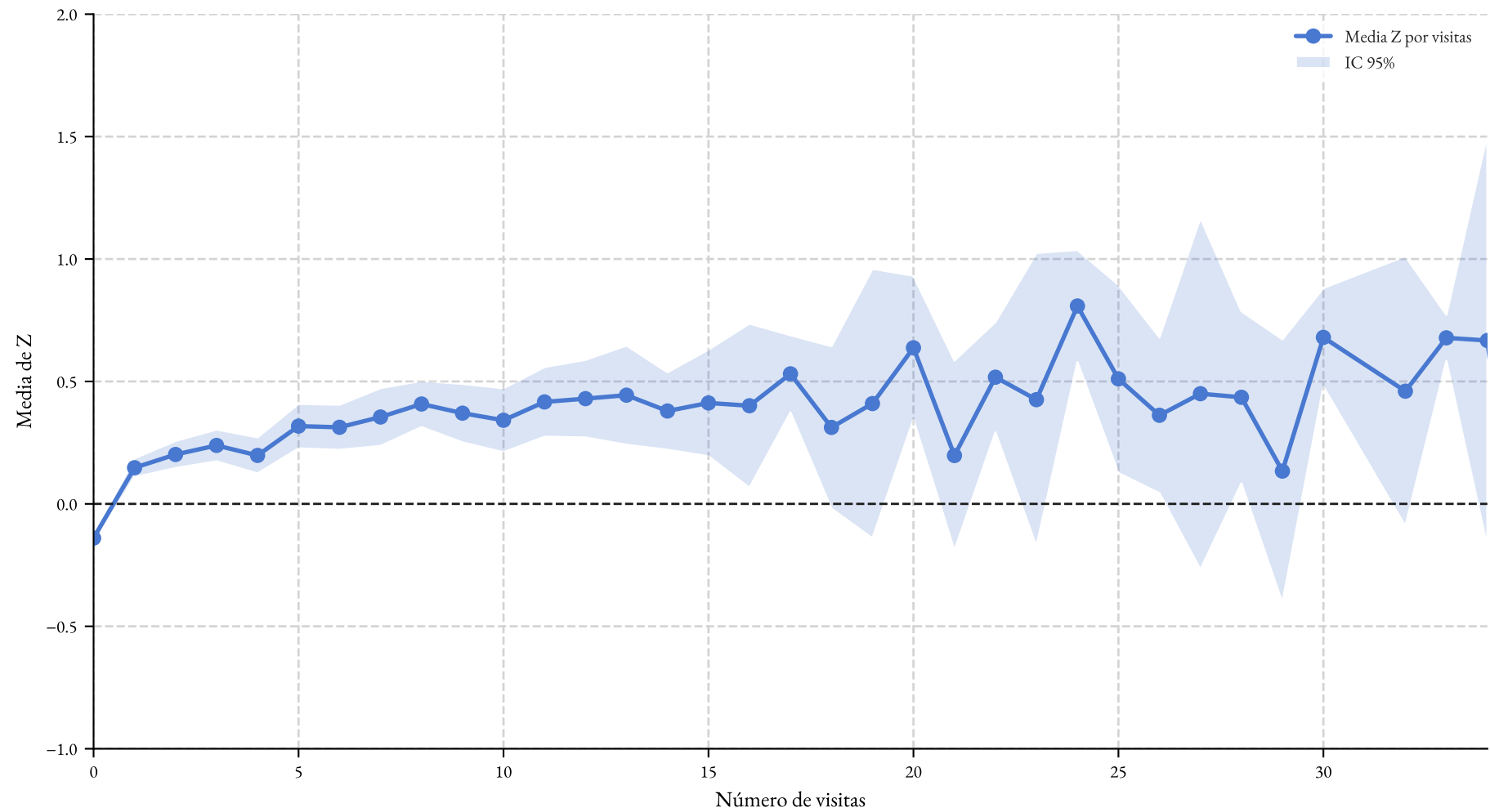
Z Promedio por salón vs número de visitas
